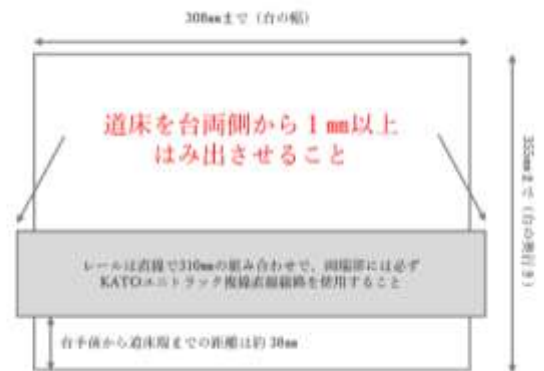
〈図 2：台を上から見た図〉
