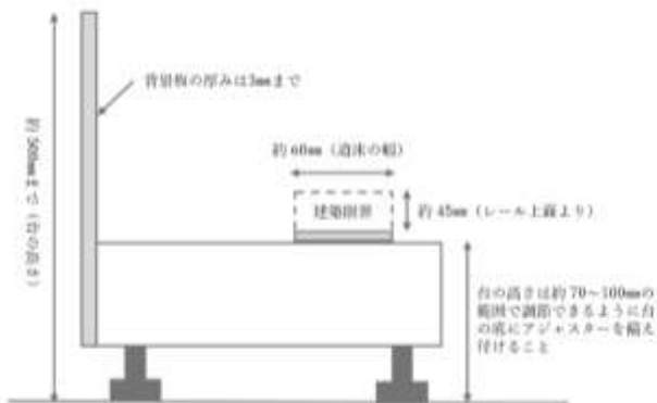
〈図 1：台を横から見た図〉
